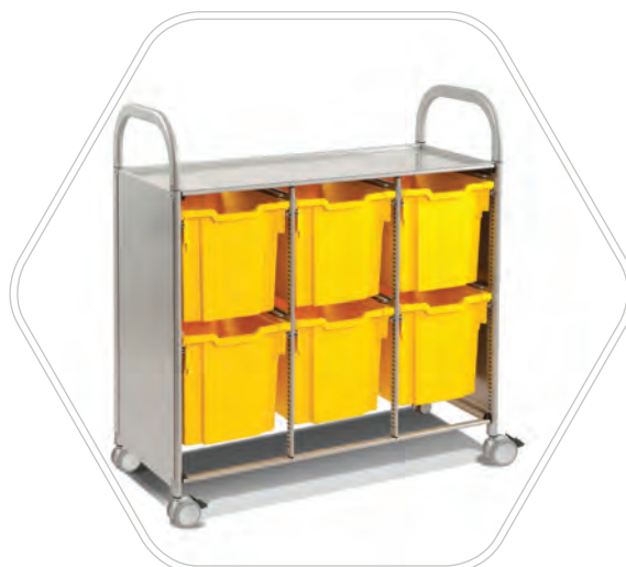
Chariot CALSET8 double colonne fourni avec 6 bacs F3 dans le coloris de votre choix. Équipé de coulisses StopSafe, il est livré avec des pieds et des roulettes avec frein. L = 1020 x p = 430 x H = 1025 mm
